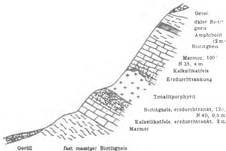
Profil durch das Magnetkiesvorkommen Schlaiten, Osttirol
